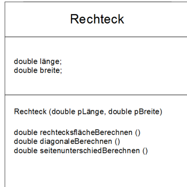
Klassendiagramm
