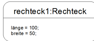
Objektdiagramm
