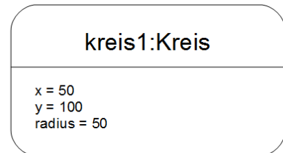
Objektdiagramm
