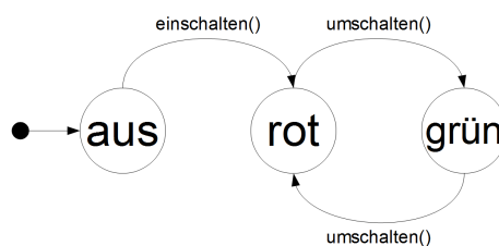
Zustandsdiagramm
