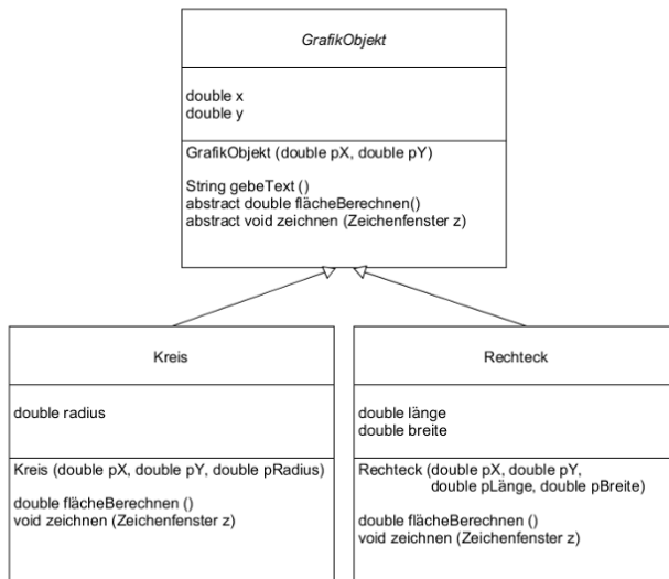
Klassendiagramm mit Vererbung
